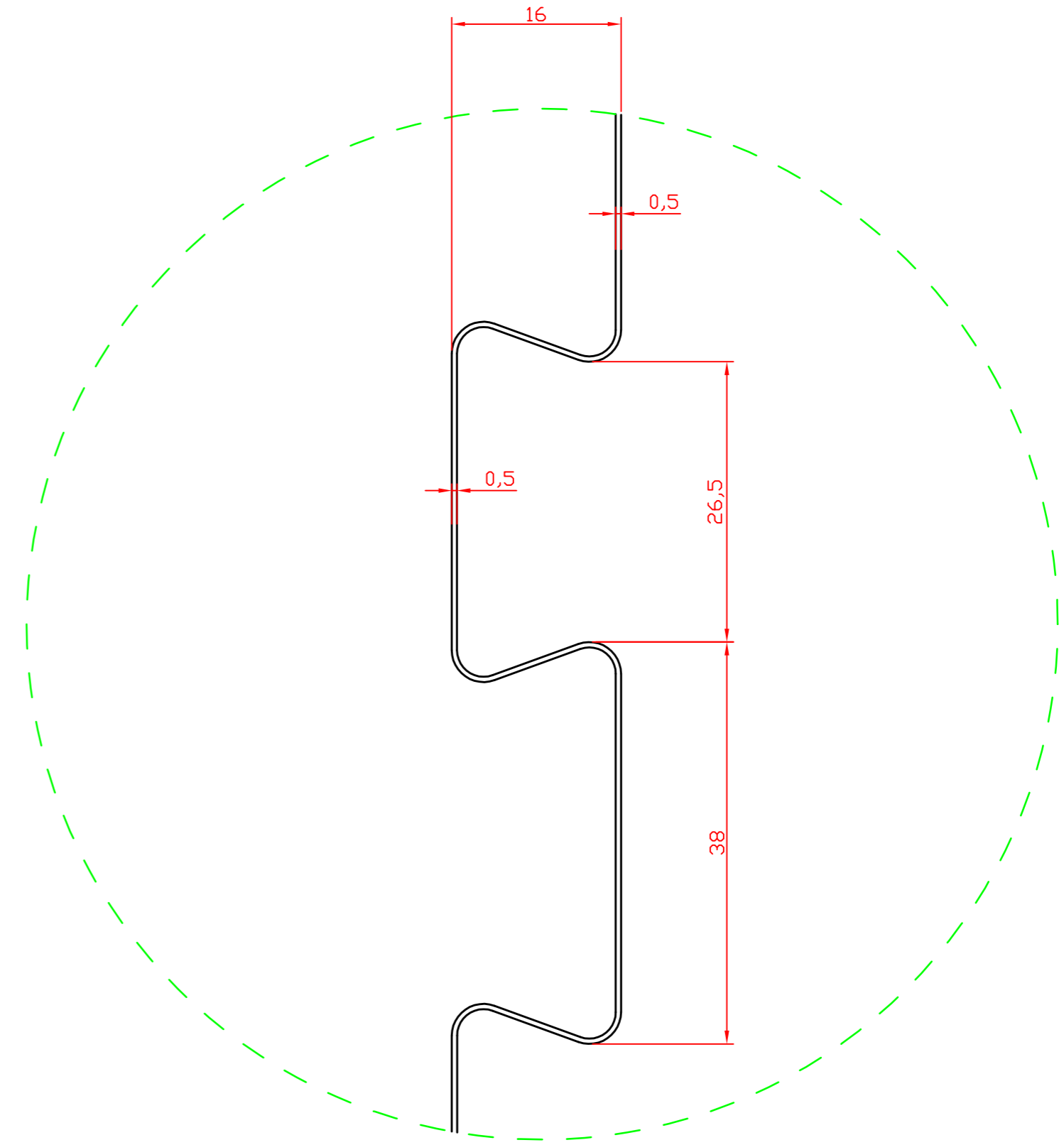
Detail Schaal 2:1
